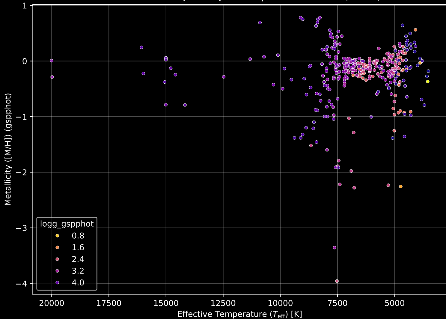
APOGEE DR17 Field: [150+00] Stellar Population Parameters (n= 385)
